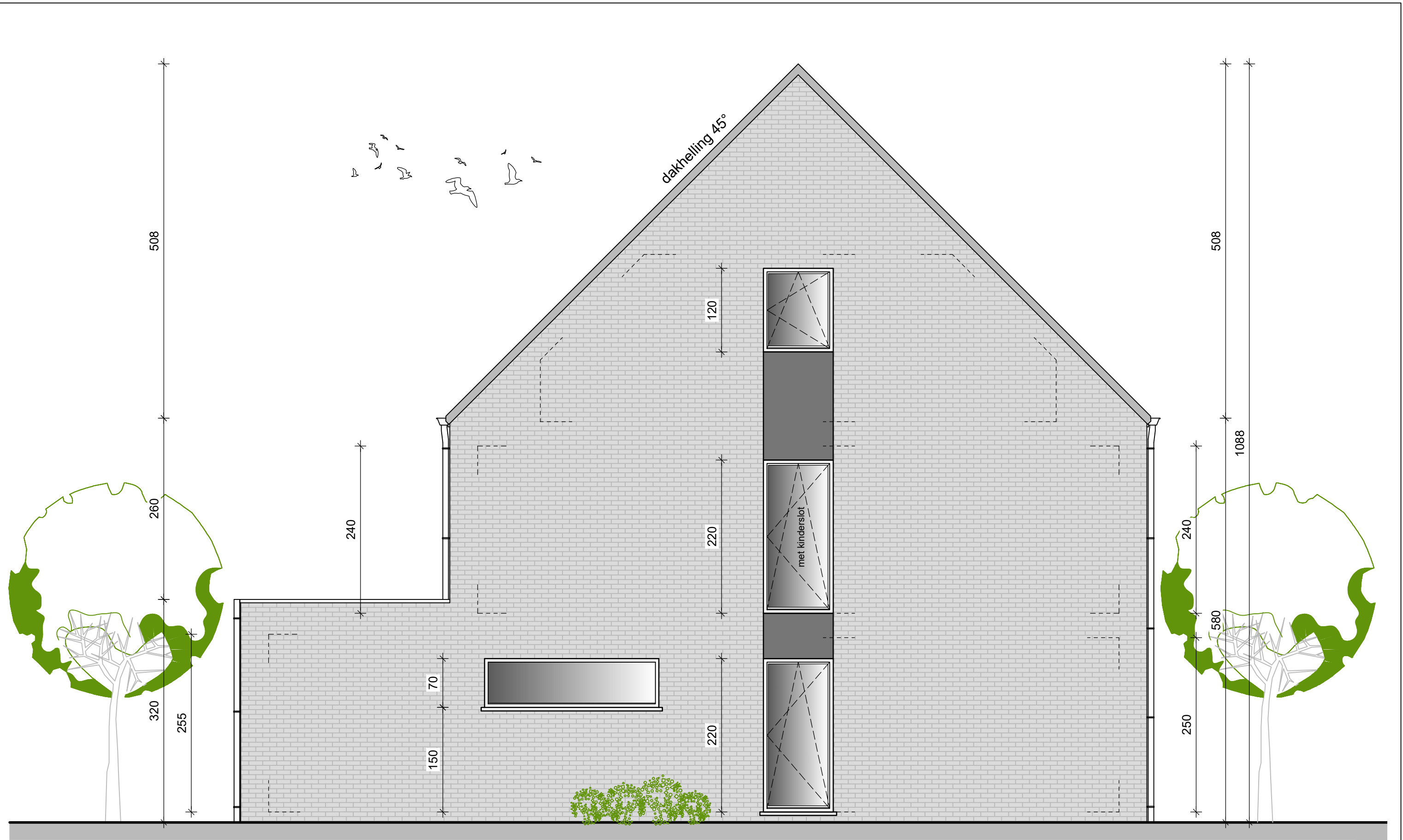
zijgevel links
