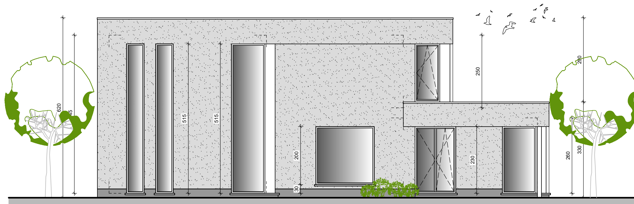
zijgevel rechts
