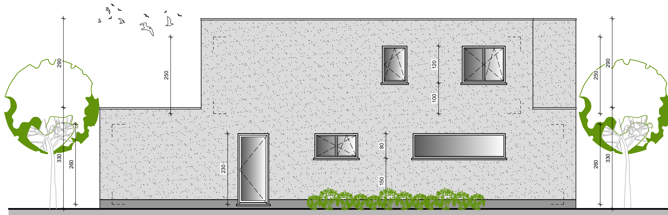
zijgevel links
