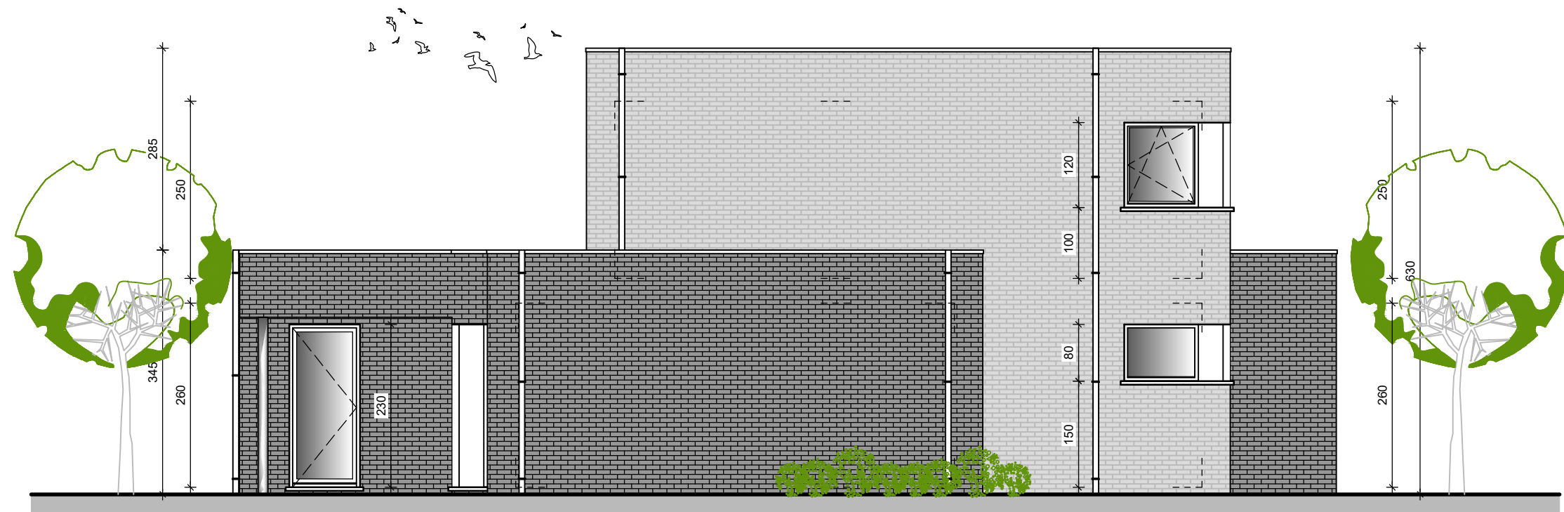
zijgevel links
