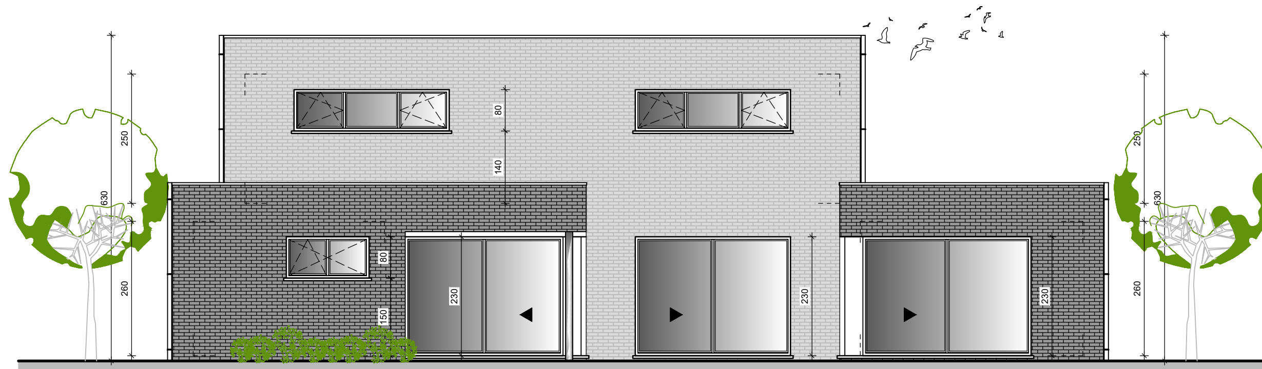
achtergevel
