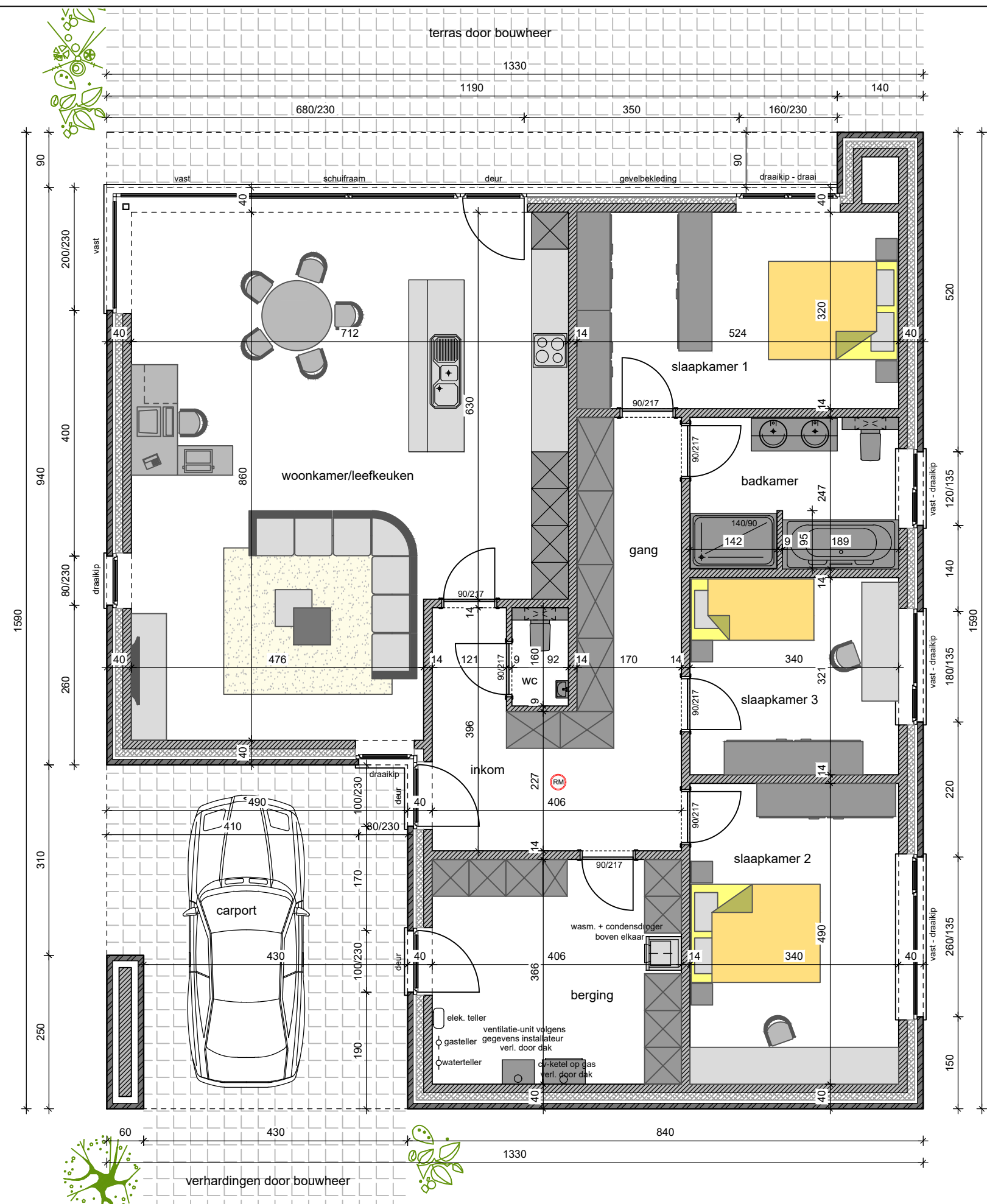
plan gelijkvloers
