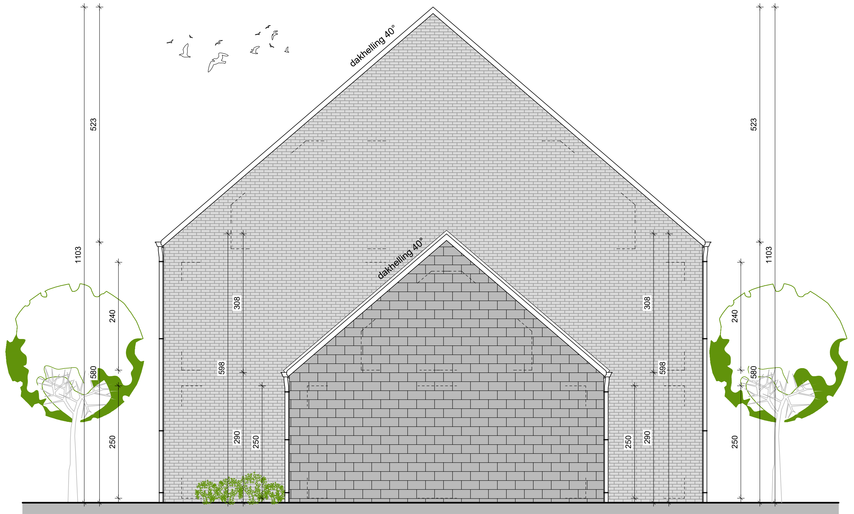
zijgevel rechts
