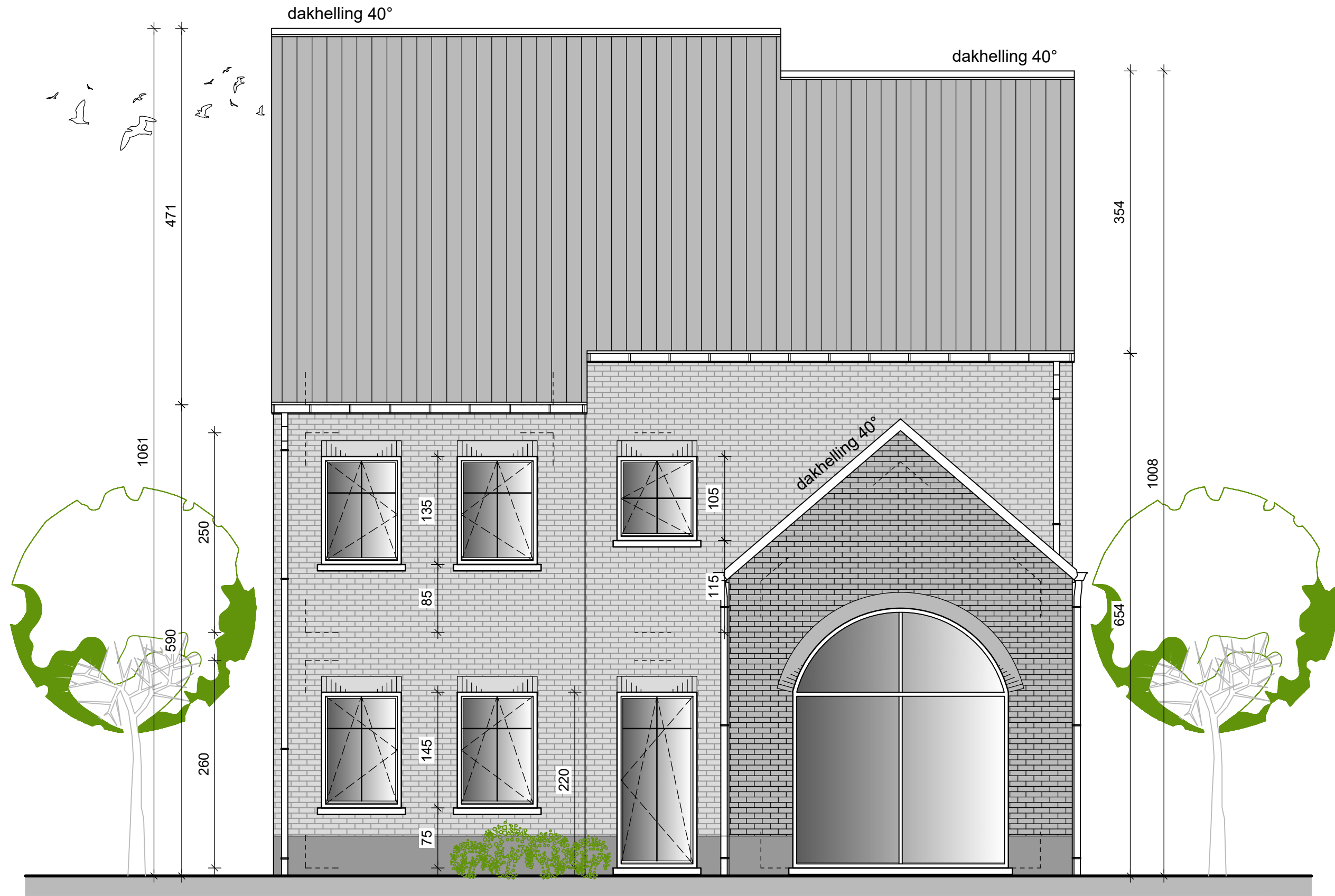
achtergevel
