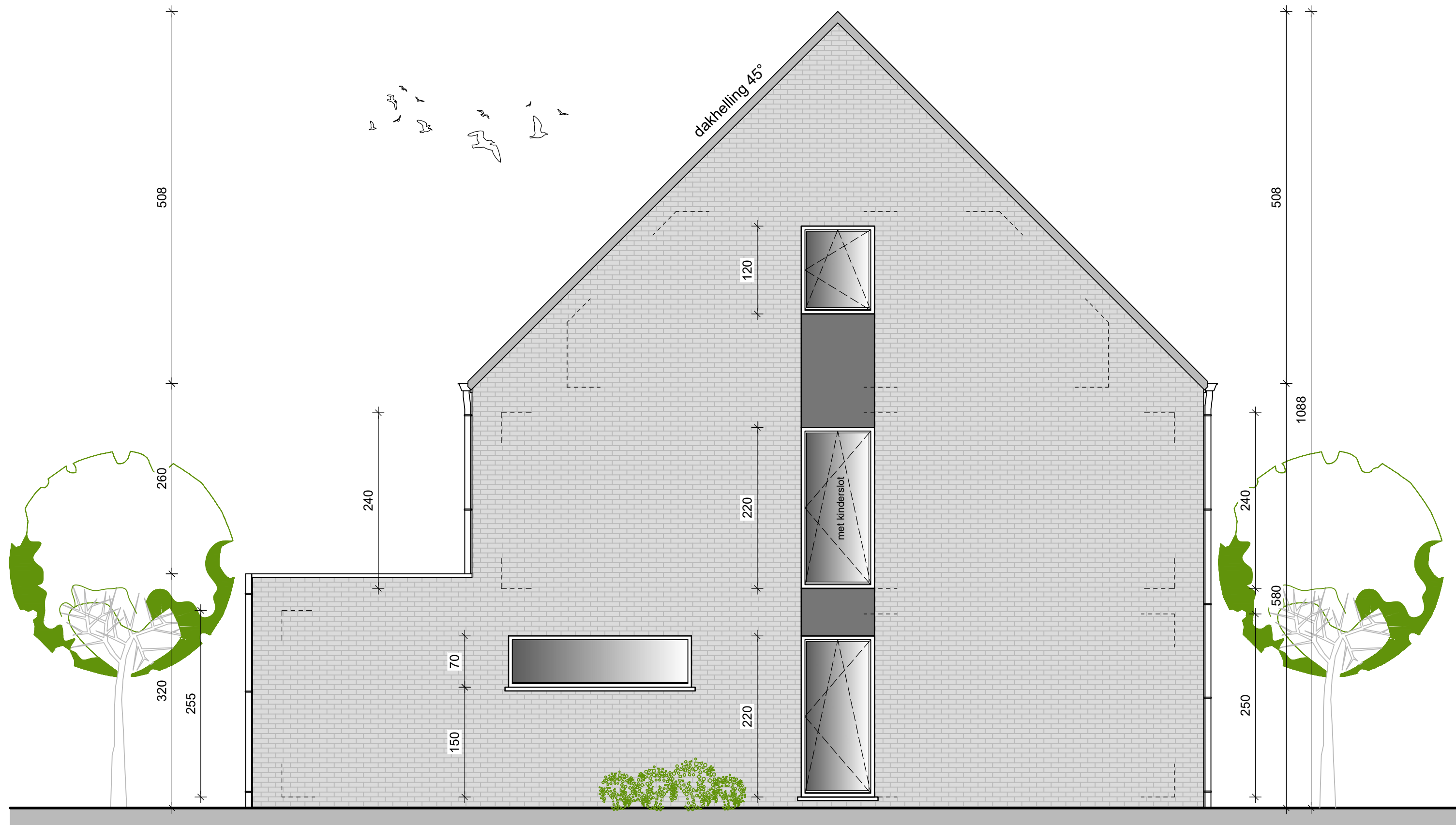
zijgevel links
